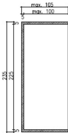
PIANTA
