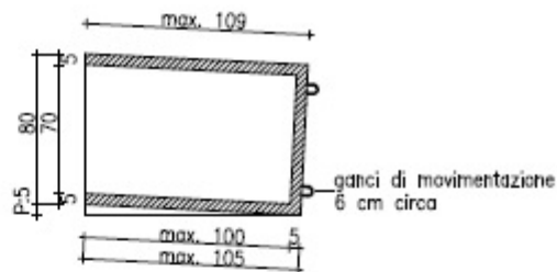
SEZIONE
